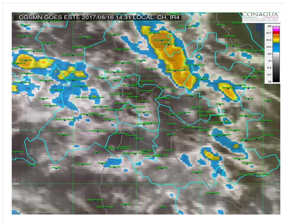
Imagen de satélite en canal infrarrojo de las 14:31 hora local
